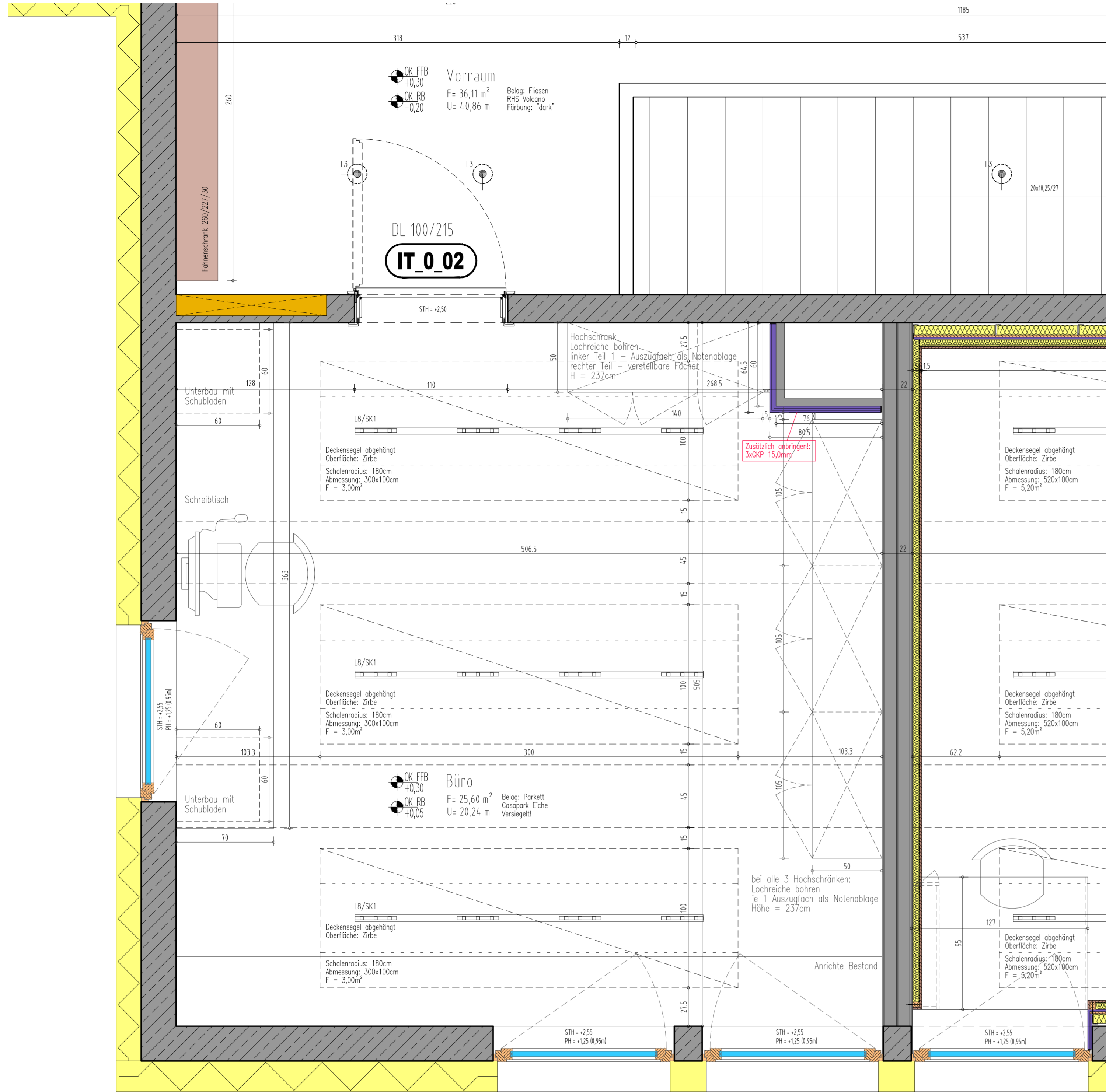
Grundriss EG - Büro M1:20
